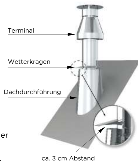
Bild 23: Dachdurchführung
