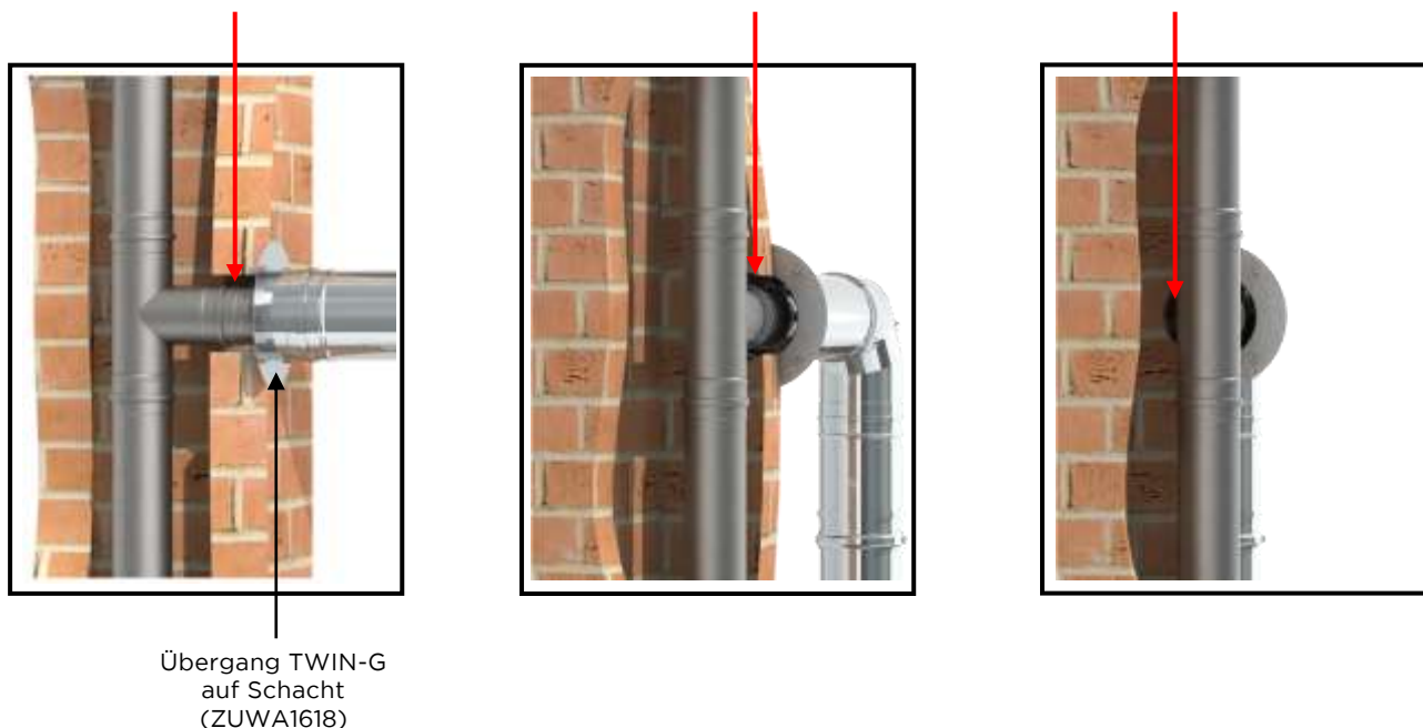
Bild 36: Ringspalt bei Übergang konzentrische Verbindungsleitung auf EW-FU im Schacht
