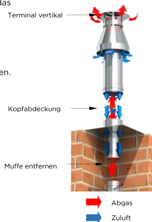
Bild 40: Terminal senkrecht
