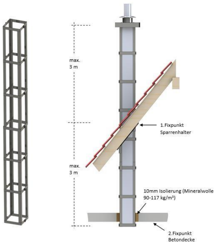
(Darstellung ohne Schachtverkleidung/ Einblechung)
