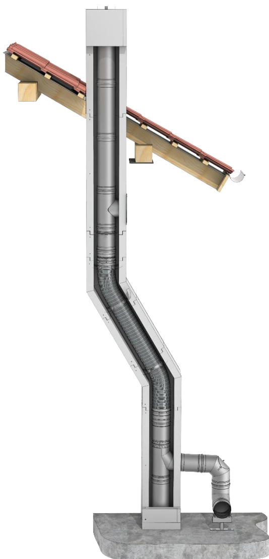
Schrägföhrung mit LINE-F
