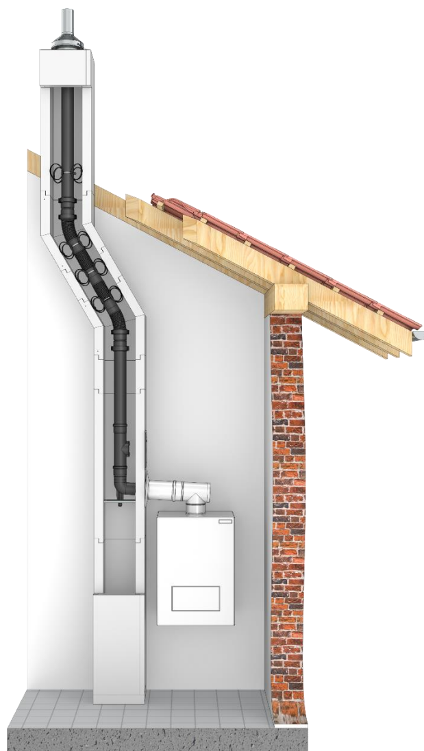
Schrägföhrung mit EW-PP-FLEX
